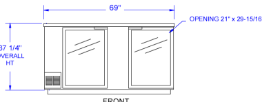
BB68G
