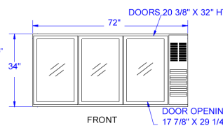
BB72G/BB72GY
